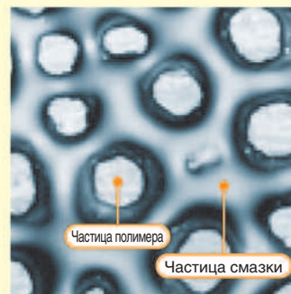
После пропитывания смазкой (Структура капиллярной смазки) Смазка удерживается в полостях между частицами полимера.
