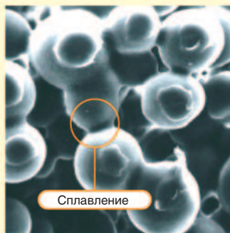
До пропитывания смазкой Соединенные сплавлением частицы полимера.
